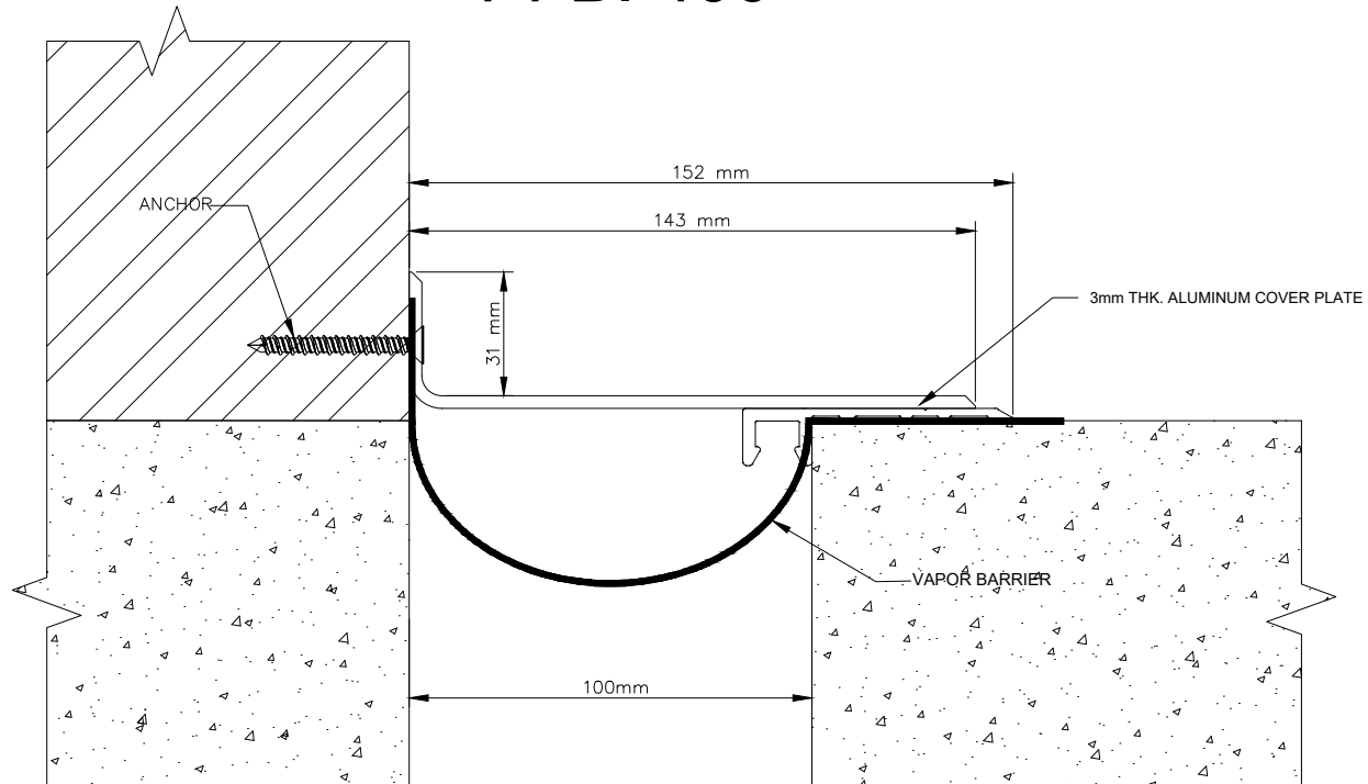
PFBIW 400
