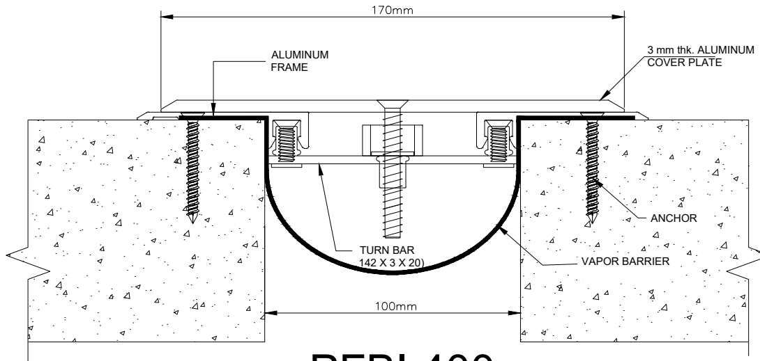
PFBI 400
