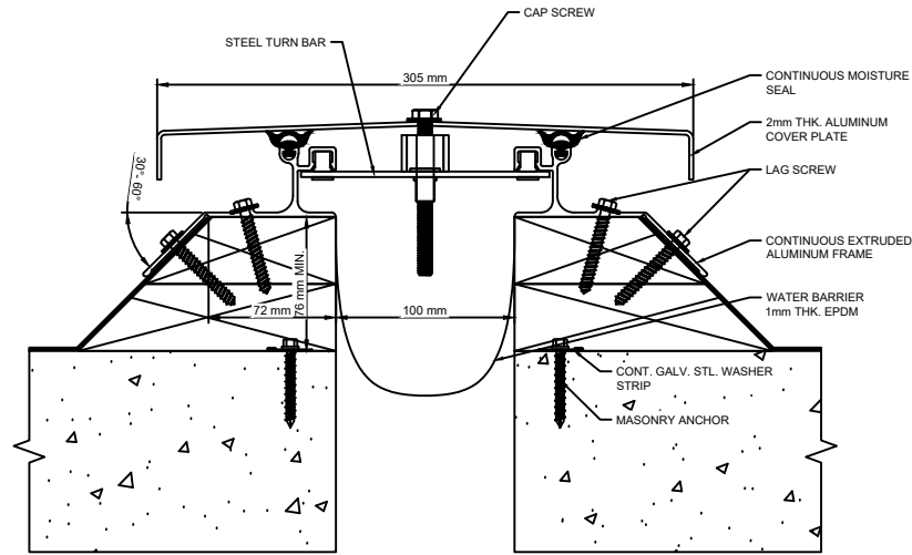
PRJ-400
