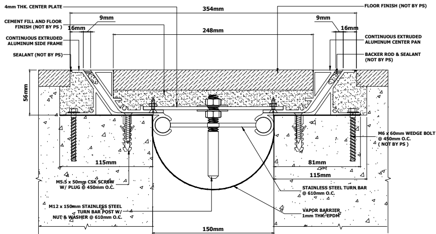
PSR - 600
