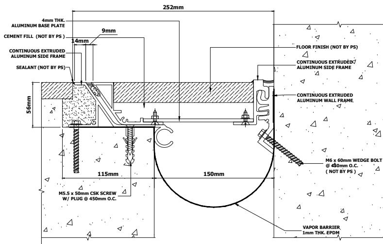
PSRW - 600
