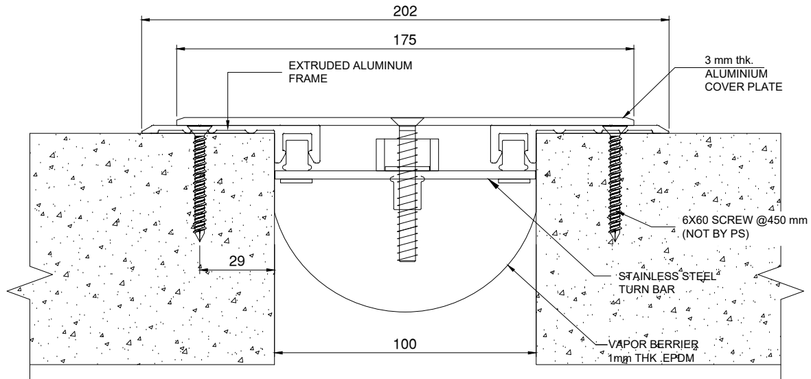
PFBI-400
