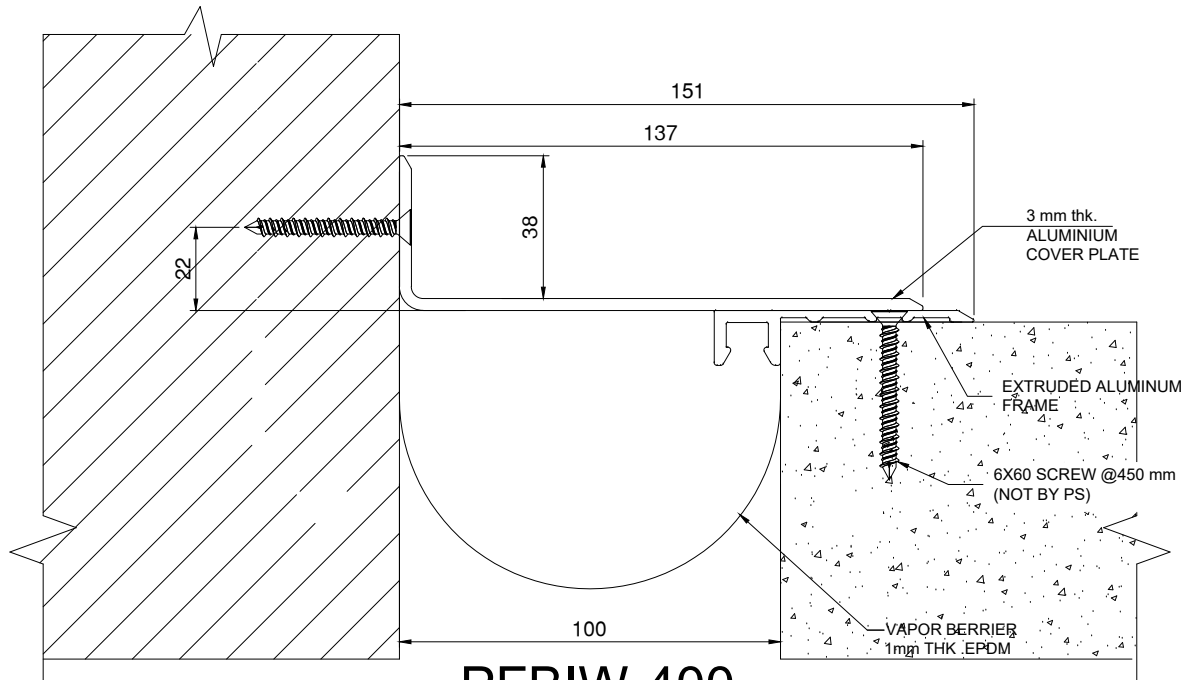
PFBIW-400
